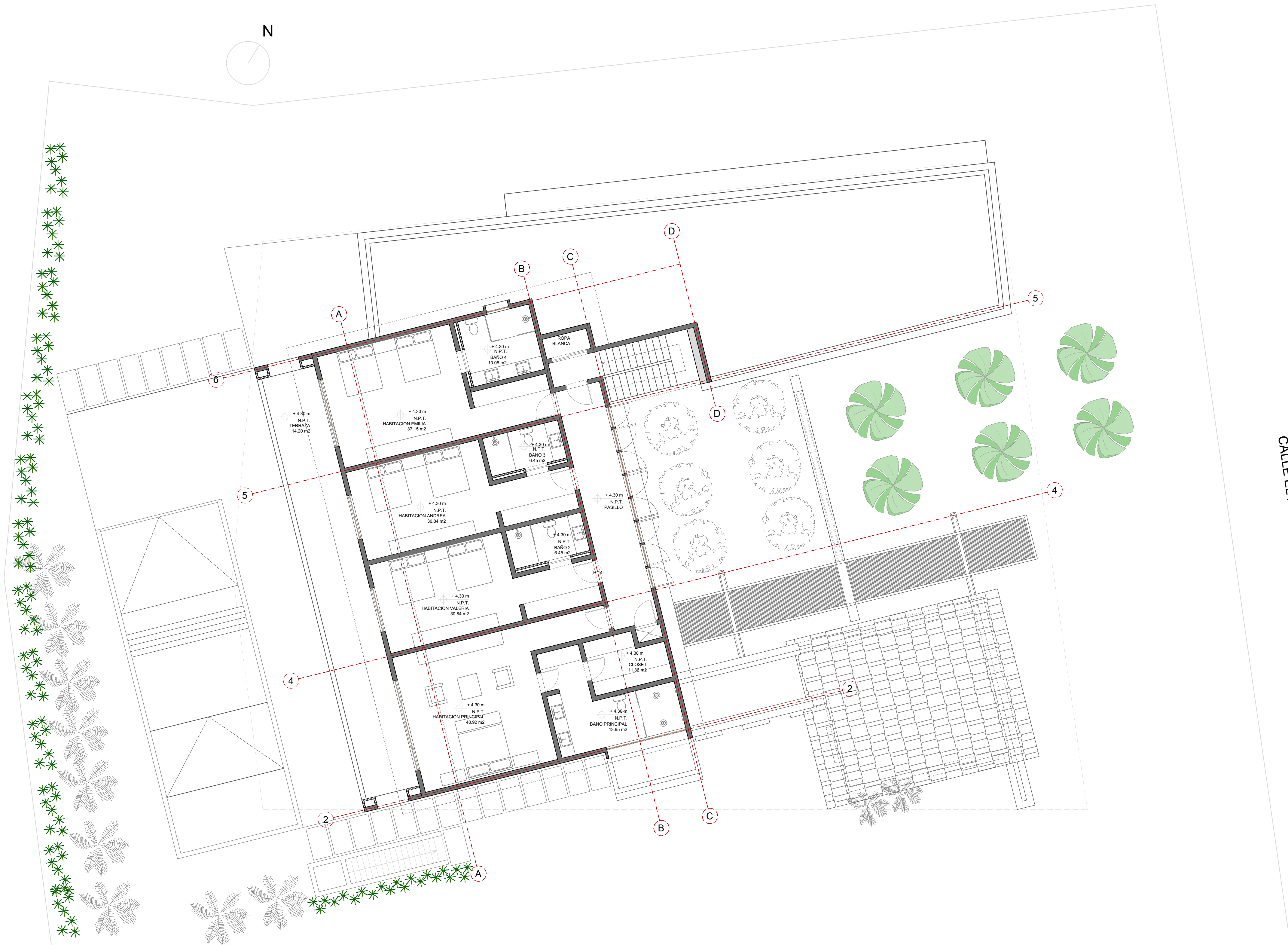
PLANTA SEGUNDO NIVEL ESC. 1:100
