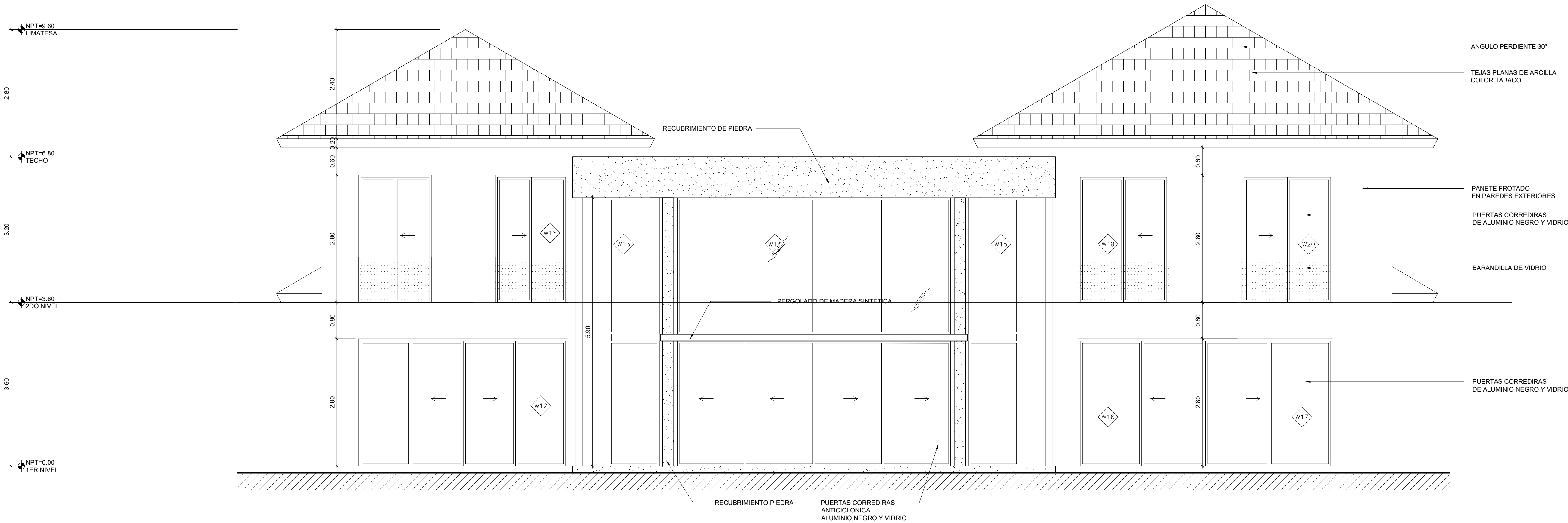
2 A-200 ELEVACION POSTERIOR E2 ESCALA 1:50
