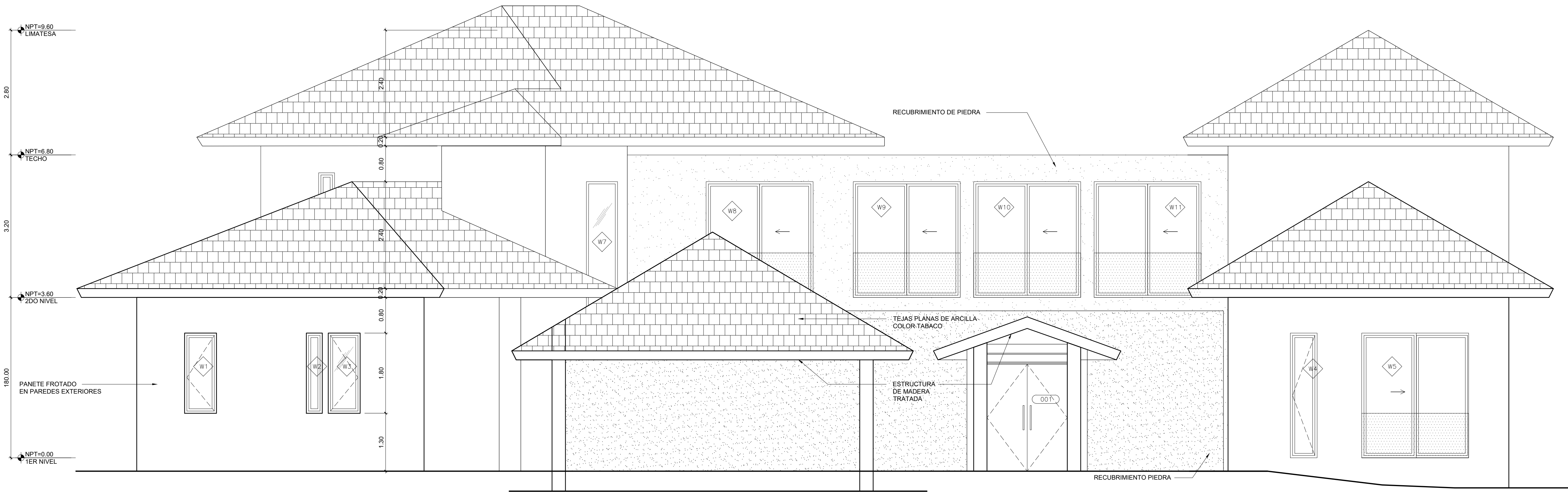
1 A-200 ELEVACION FRONTAL E1 ESCALA 1:50
