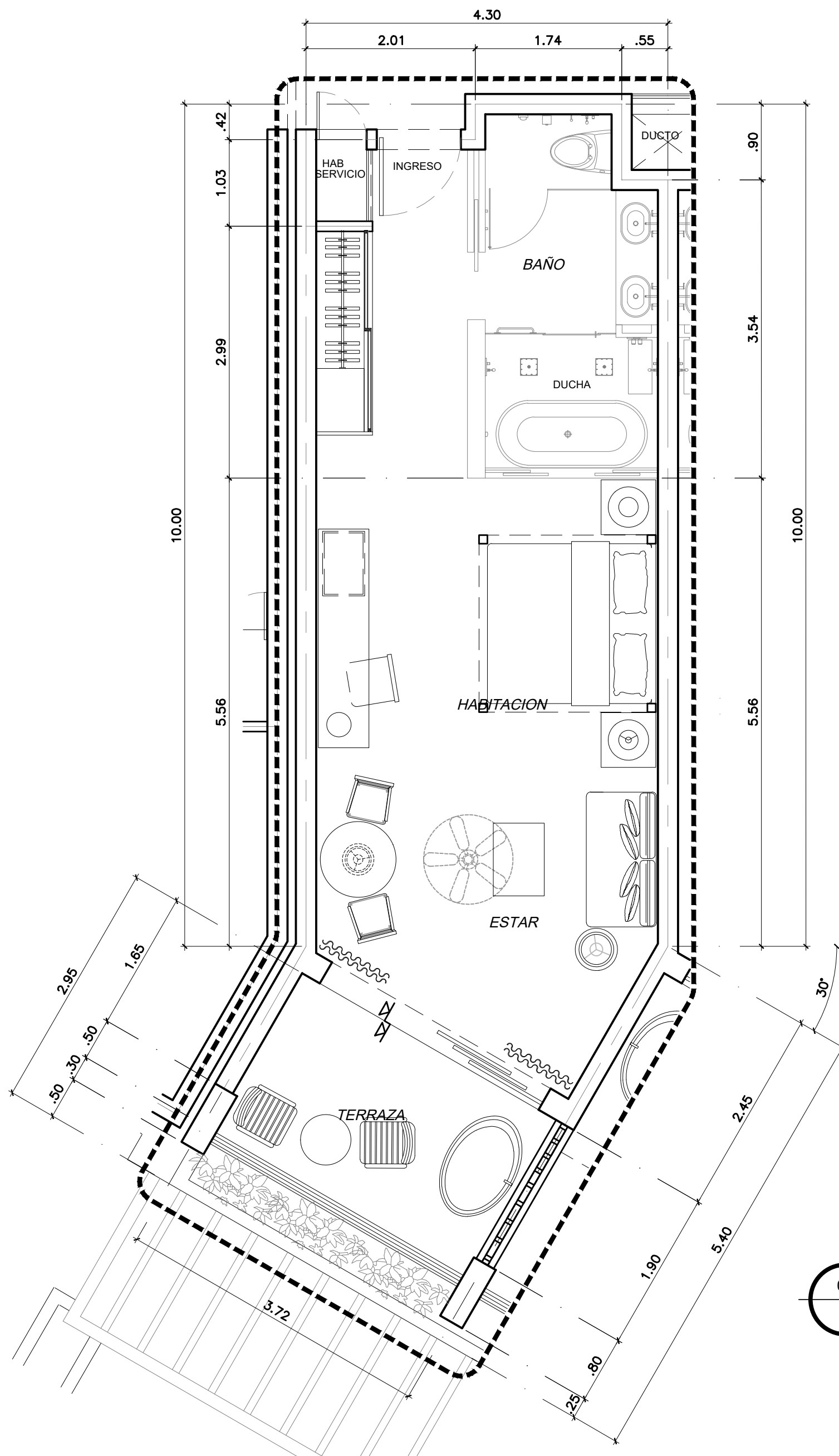
04 HABITACION JUNIOR SUITE DIAGONAL PREFERRED ESQ. "B" N1 ESC. 1:50 METROS
