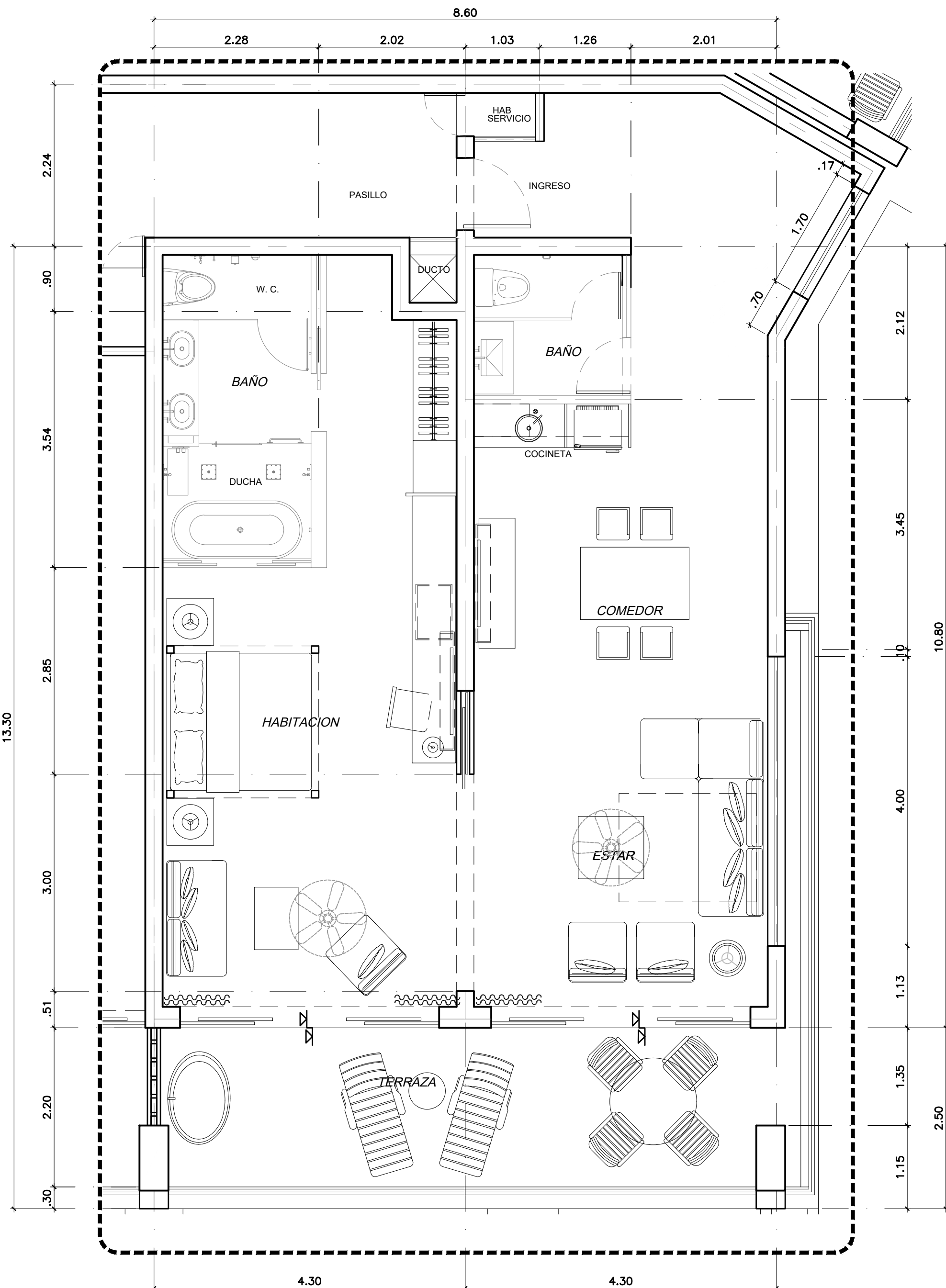
02 HABITACION MASTER RECTA PREFERRED ESQ. N1 ESC. 1:50 METROS
