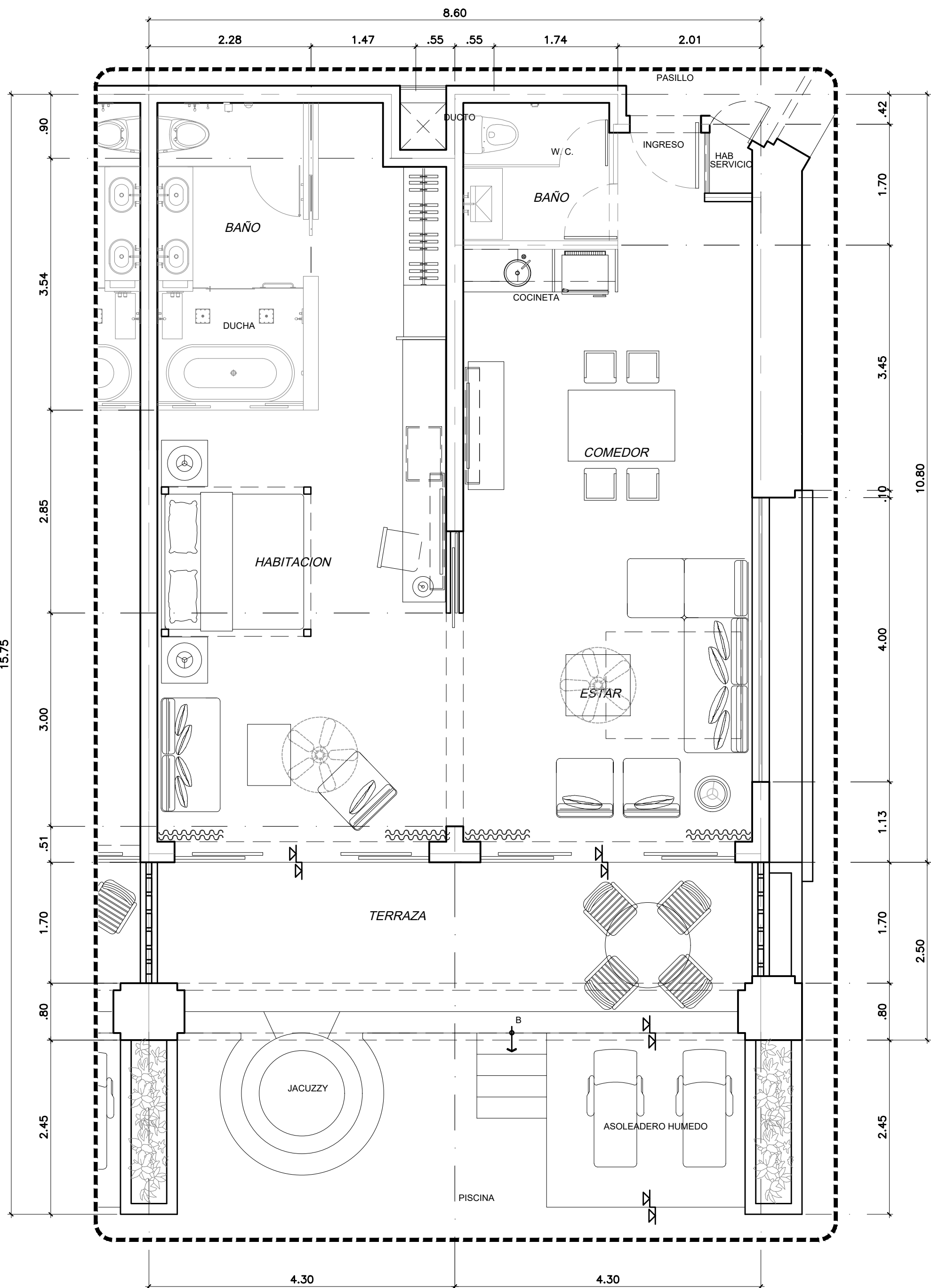
01 HABITACION MASTER RECTA PREFERRED PB ESQUINERA ESC. 1:50 METROS
