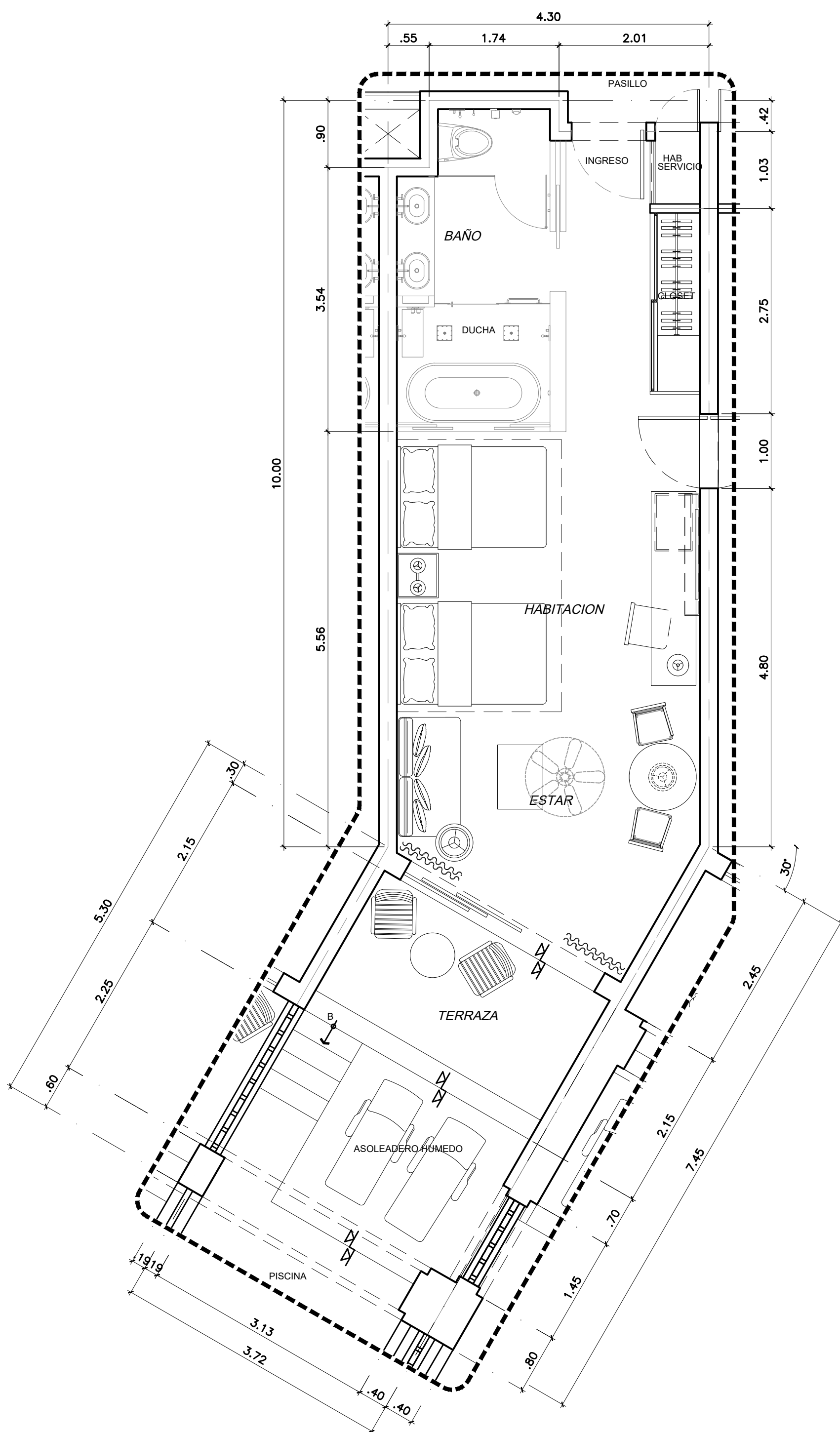
02 HABITACION JUNIOR SUITE DIAGONAL PREFERRED PB "B" INTERCOM ESC. 1:50 METROS
