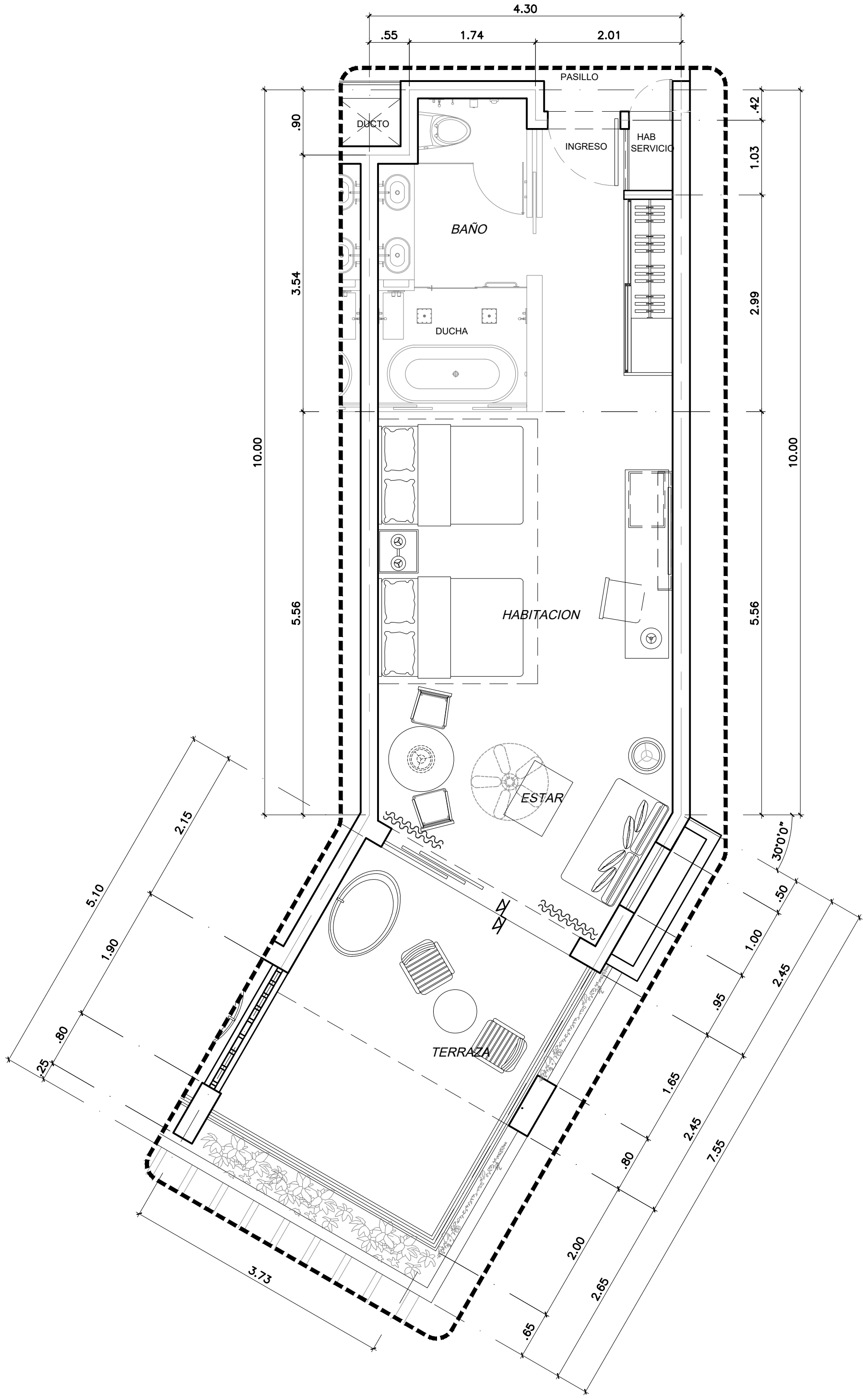
01 HABITACION JUNIOR SUITE DIAGONAL PREFERRED ESQ. N1 ESC. 1:50 METROS
