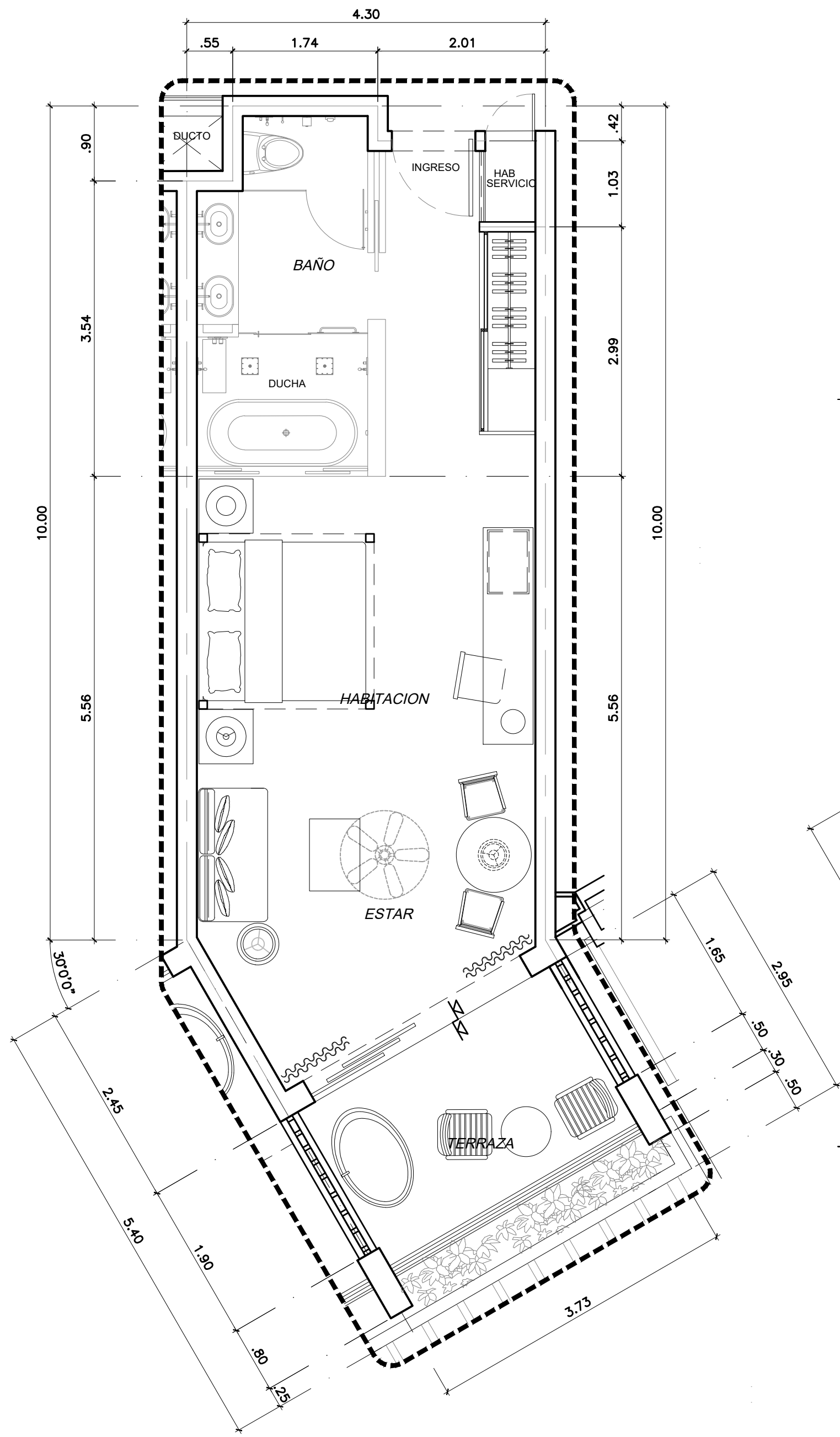
HABITACION JUNIOR SUITE DIAGONAL PREFERRED ESQ. "B" N1 ESC. 1:50 METROS
