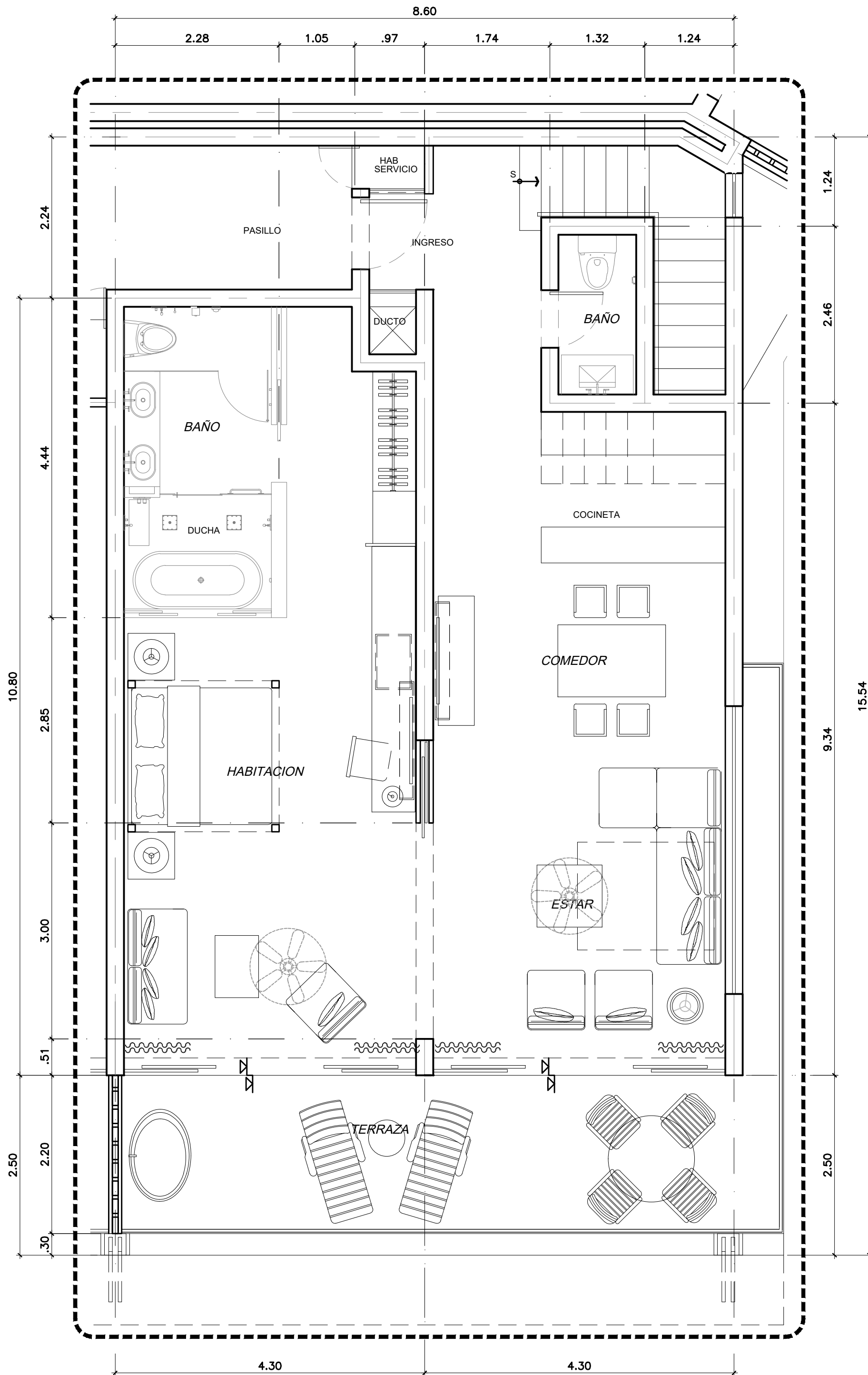
03 MASTER SUITE RECTA PREFERRED ESQ. B TECHO N2 ESC. 1:50 METROS
