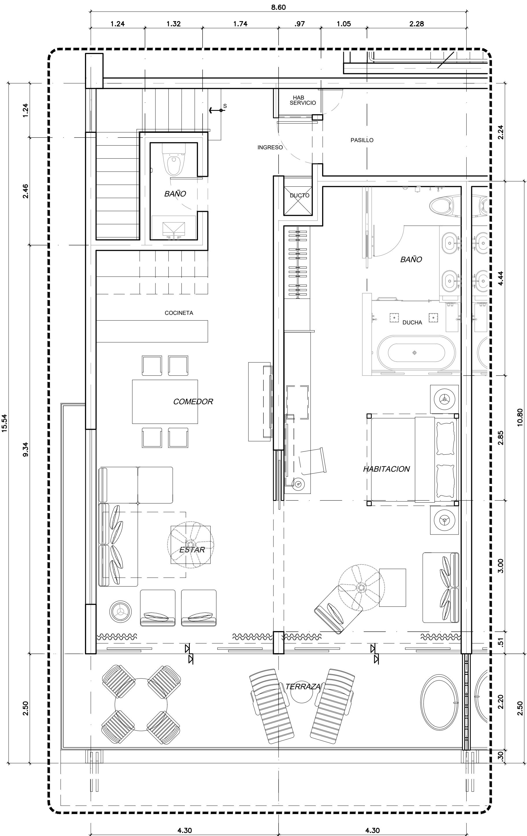
01 HABITACION MASTER RECTA PREFERRED ESQ. TECHO N2 ESC. 1:50 METROS
