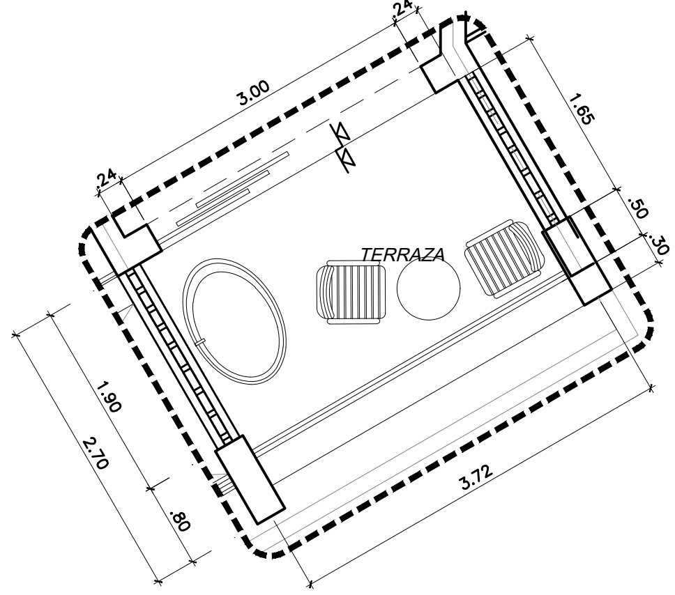
HABITACION JUNIOR SUITE DIAGONAL PREFERRED ESQ. "B" N2 ESC. 1:50 METROS
