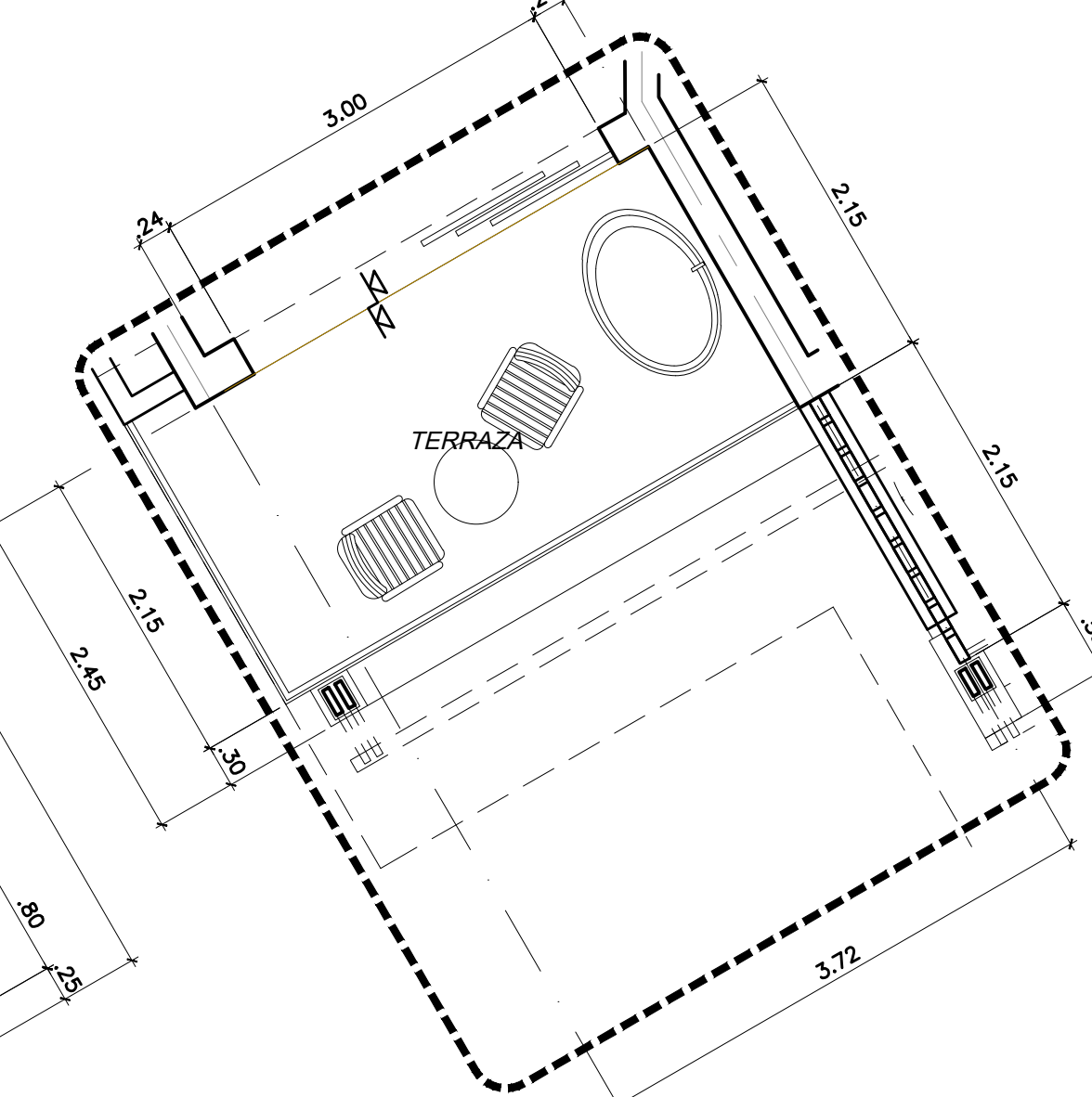
HABITACION JUNIOR SUITE DIAGONAL PREFERRED ESQ. N3 ESC. 1:50 METROS
