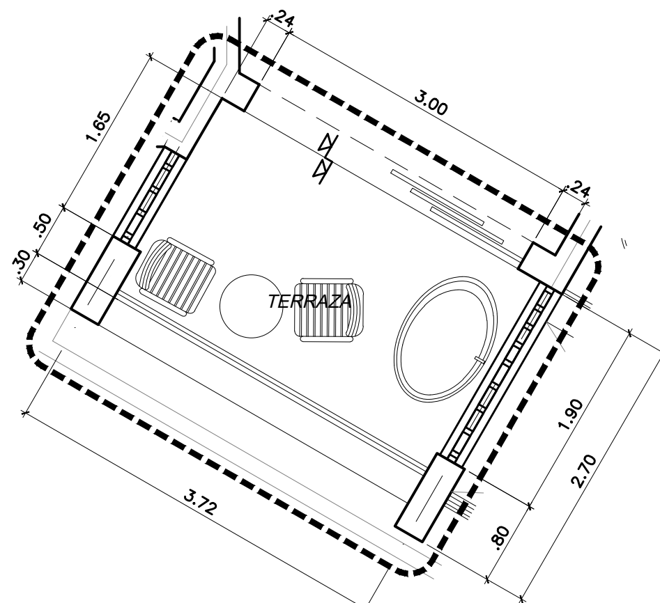
05 HABITACION JUNIOR SUITE DIAGONAL PREFERRED ESQ. "B" N2 ESC. 1:50 METROS
