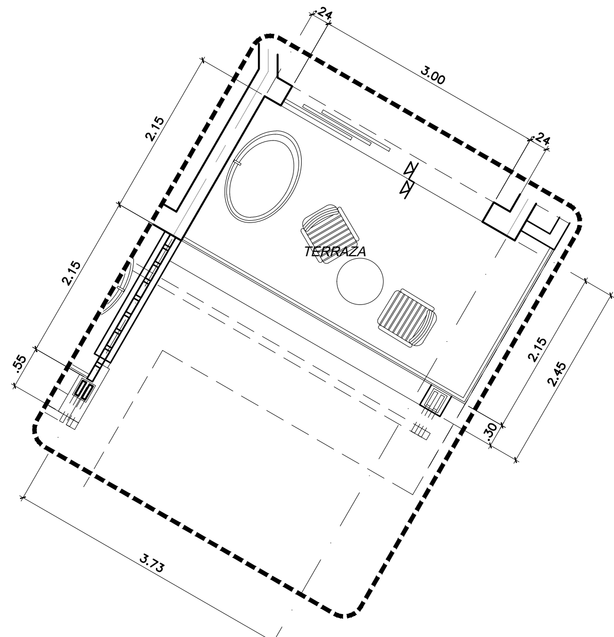
02 HABITACION JUNIOR SUITE DIAGONAL PREFERRED ESQ. N2 ESC. 1:50 METROS
