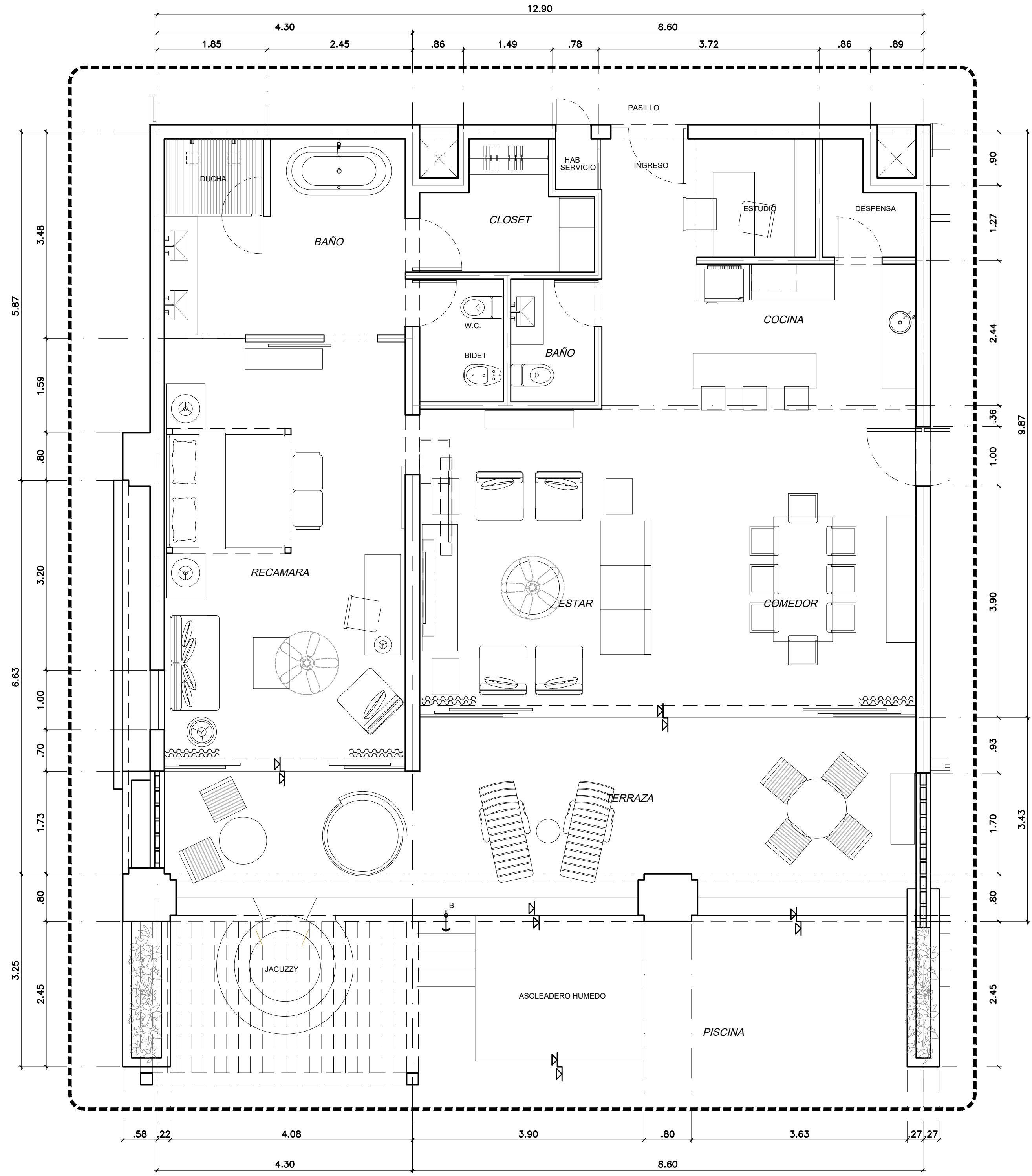
01 HABITACION PRESIDENCIAL P. B. ESC. 1:50 METROS
