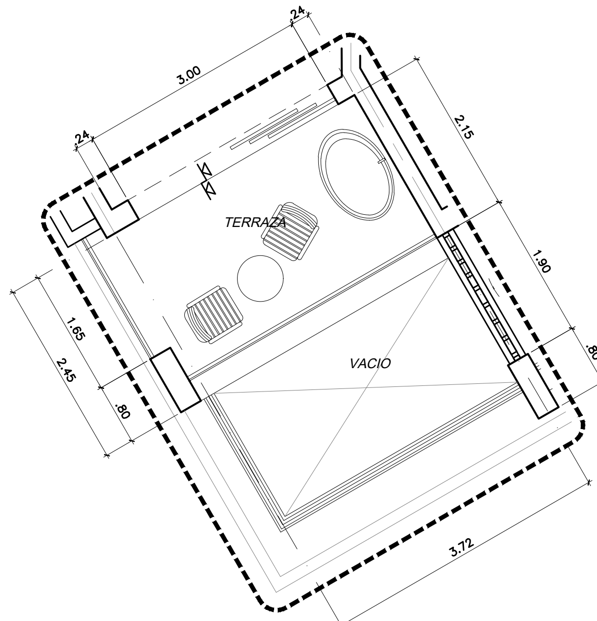
HABITACION JUNIOR SUITE DIAGONAL PREFERRED ESQ. N2 ESC. 1:50 METROS
