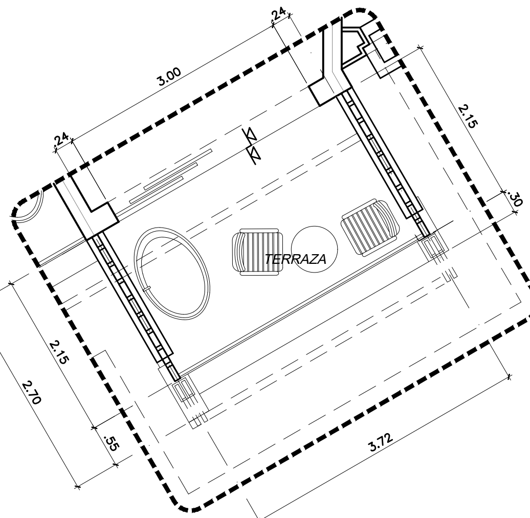
HABITACION JUNIOR SUITE DIAGONAL PREFERRED ESQ. "B" N3 ESC. 1:50 METROS
