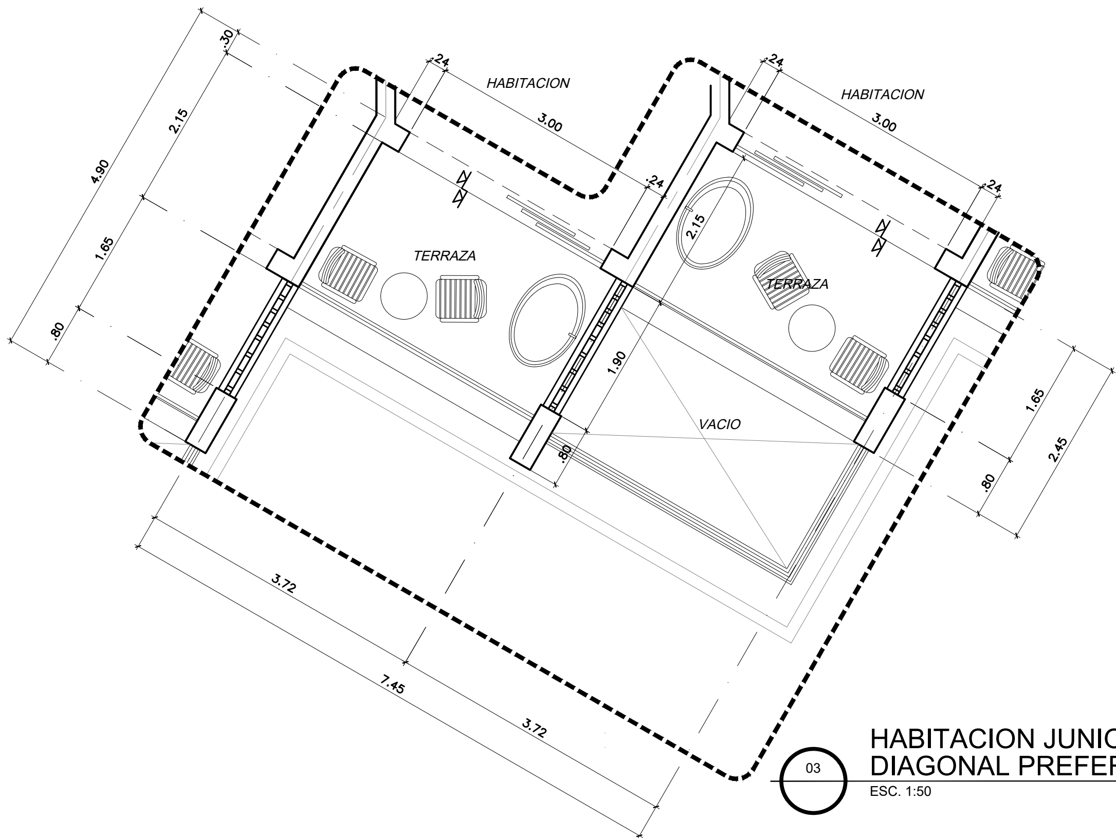
HABITACION JUNIOR SUITE DIAGONAL PREFERRED N2 ESC. 1:50 METROS
