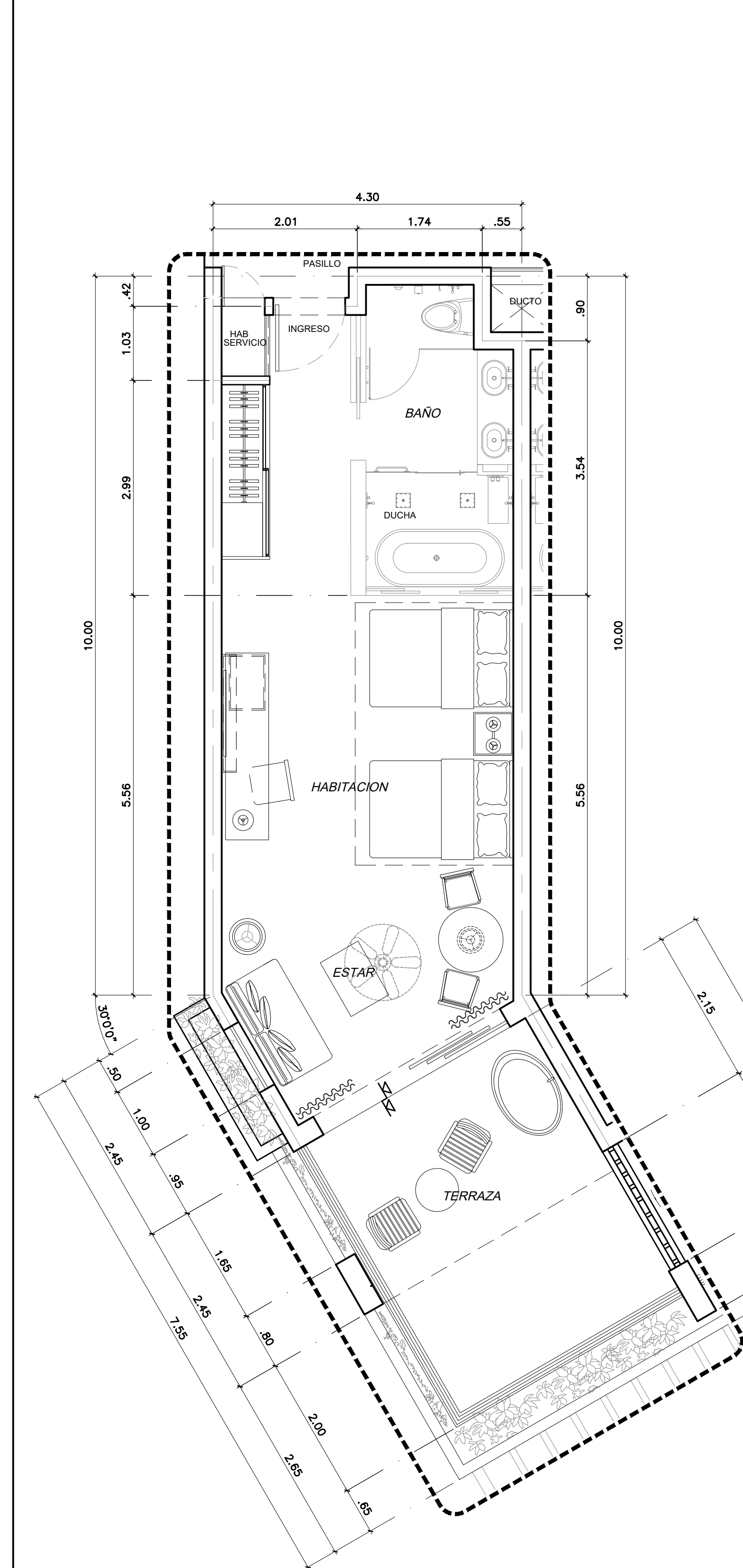
HABITACION JUNIOR SUITE DIAGONAL PREFERRED ESQ. N1 ESC. 1:50 METROS
