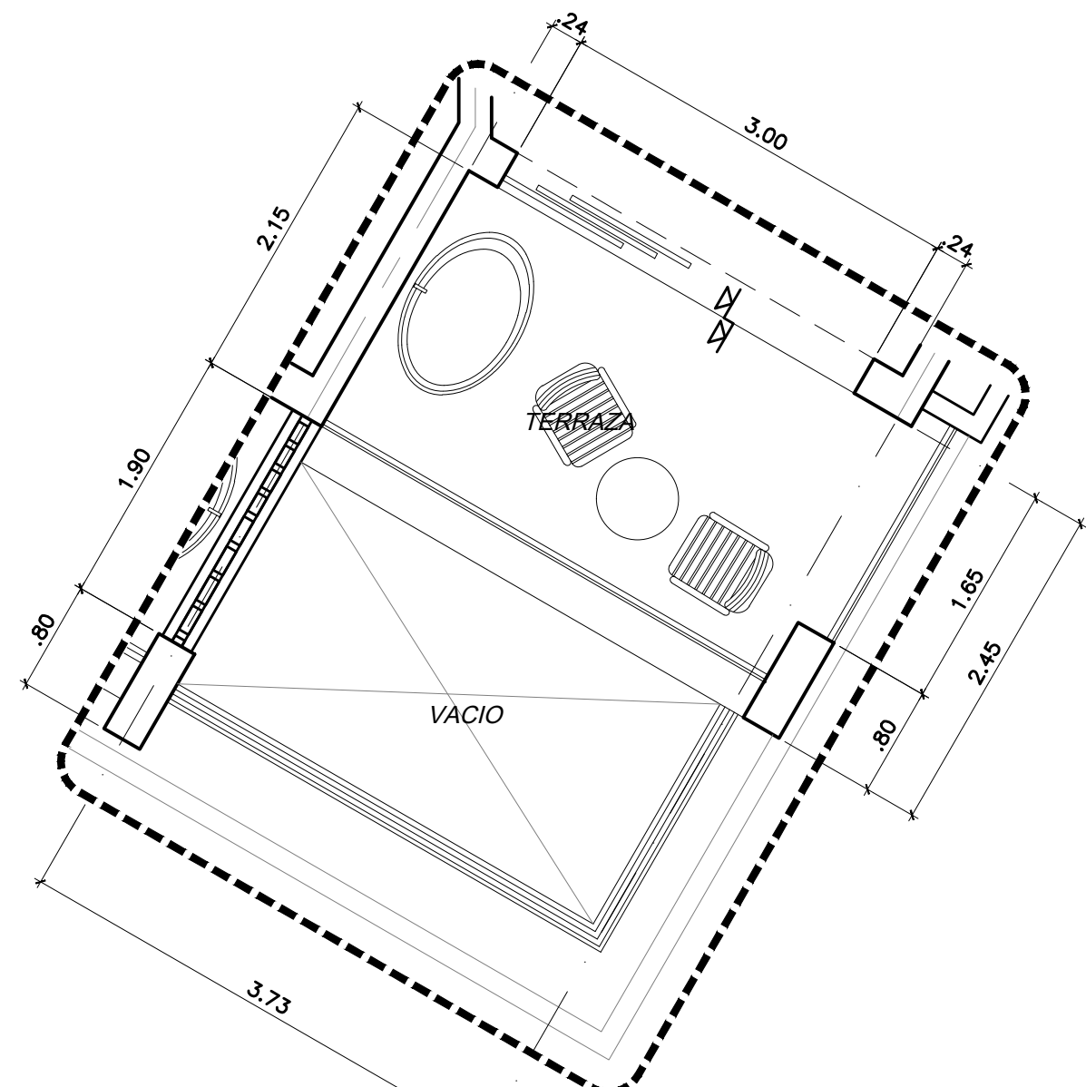
03 HABITACION JUNIOR SUITE DIAGONAL PREFERRED ESQ. N3 ESC. 1:50 METROS
